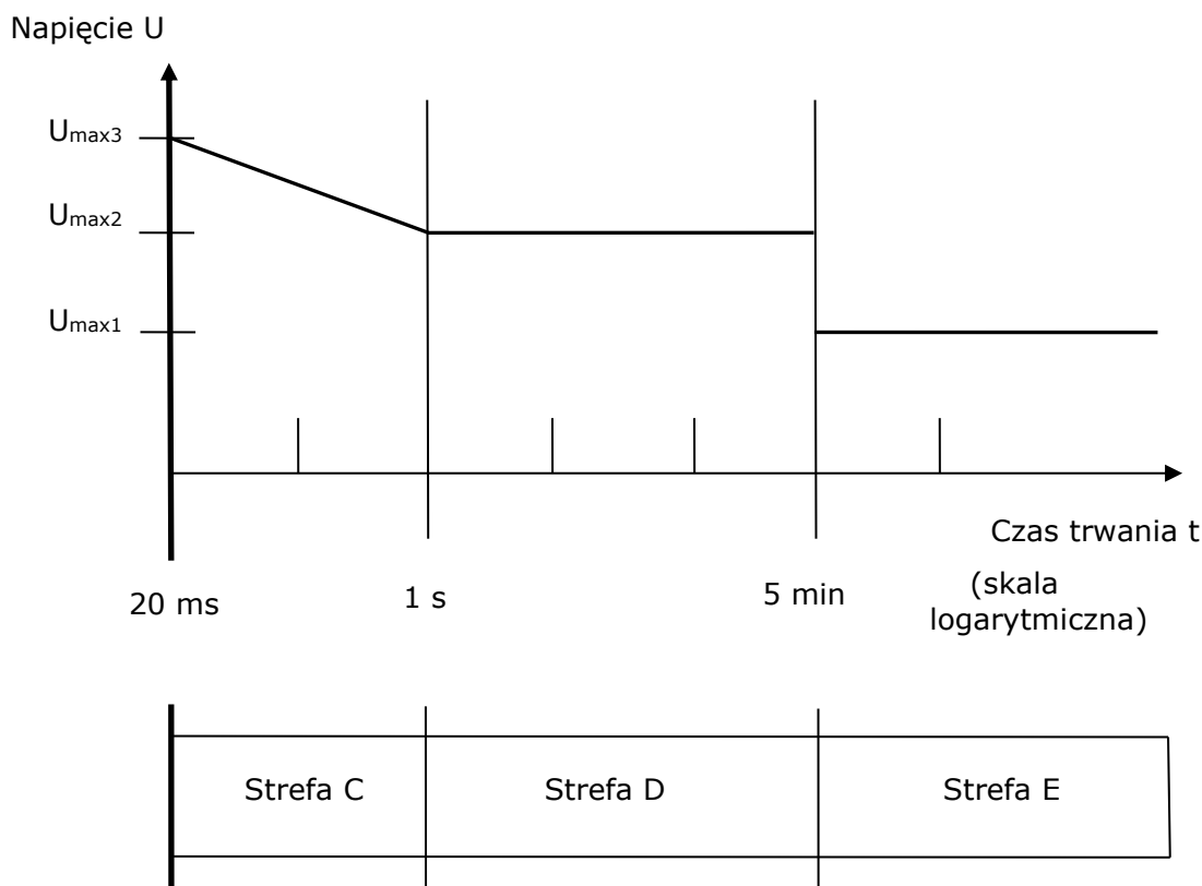
Tablica 2 – Przepięcia
