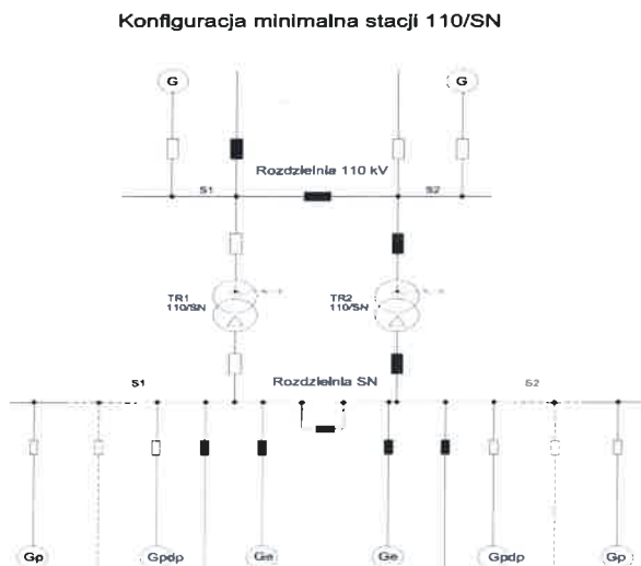
Rys.2. Konfiguracja minimalna
