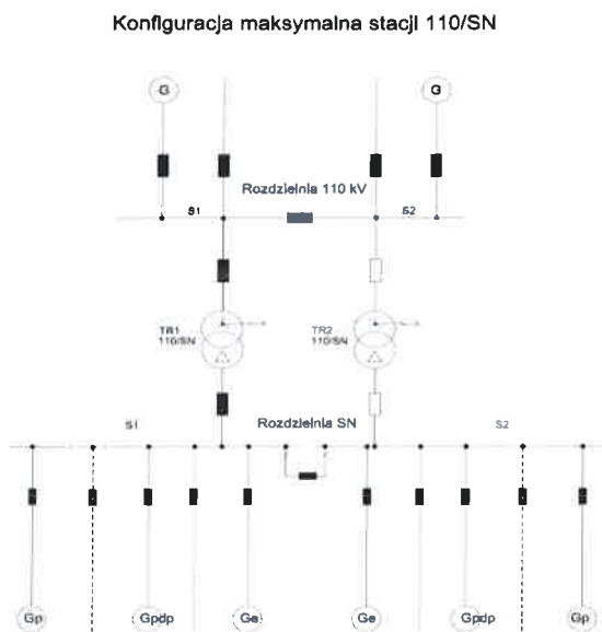
Rys.1. Konfiguracja maksymalna
